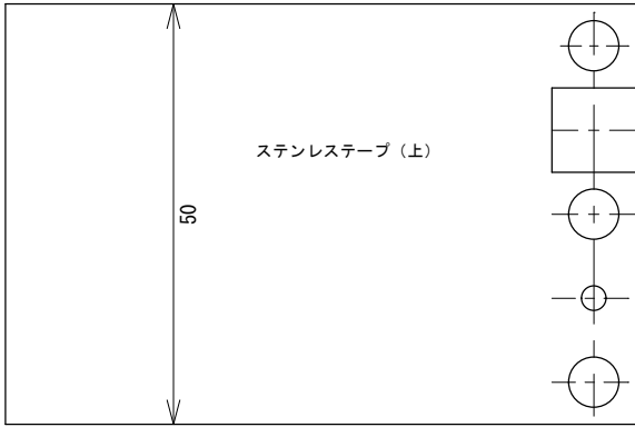
【上蓋用】 【ステンレステープ】
