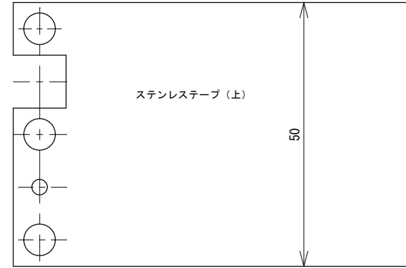
【上蓋用】 【ステンレステープ】
